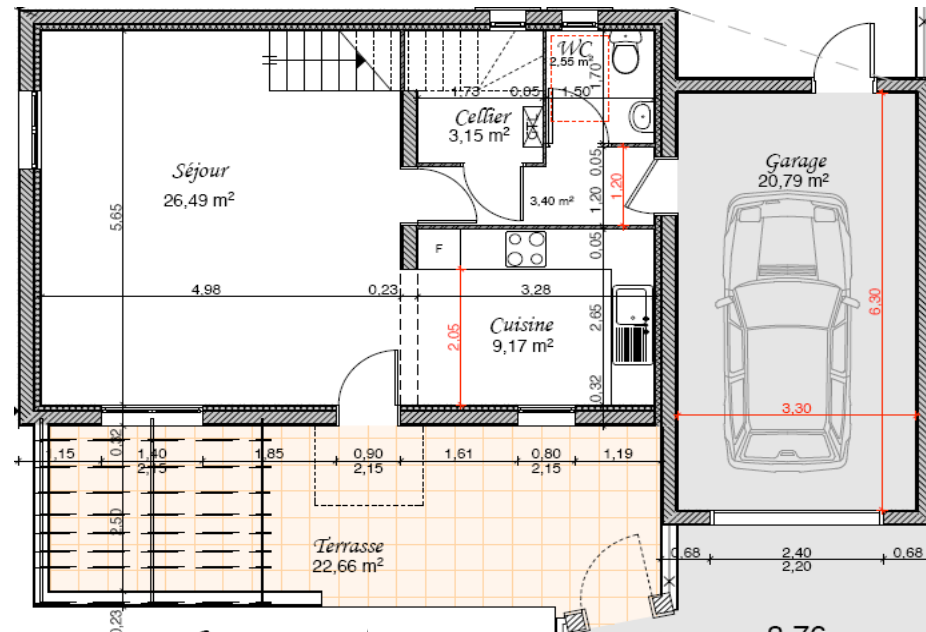
Plan RDC
